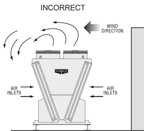
Figure 2 - Effet du vent avec le haut de l'unité plus bas que le haut du mur
